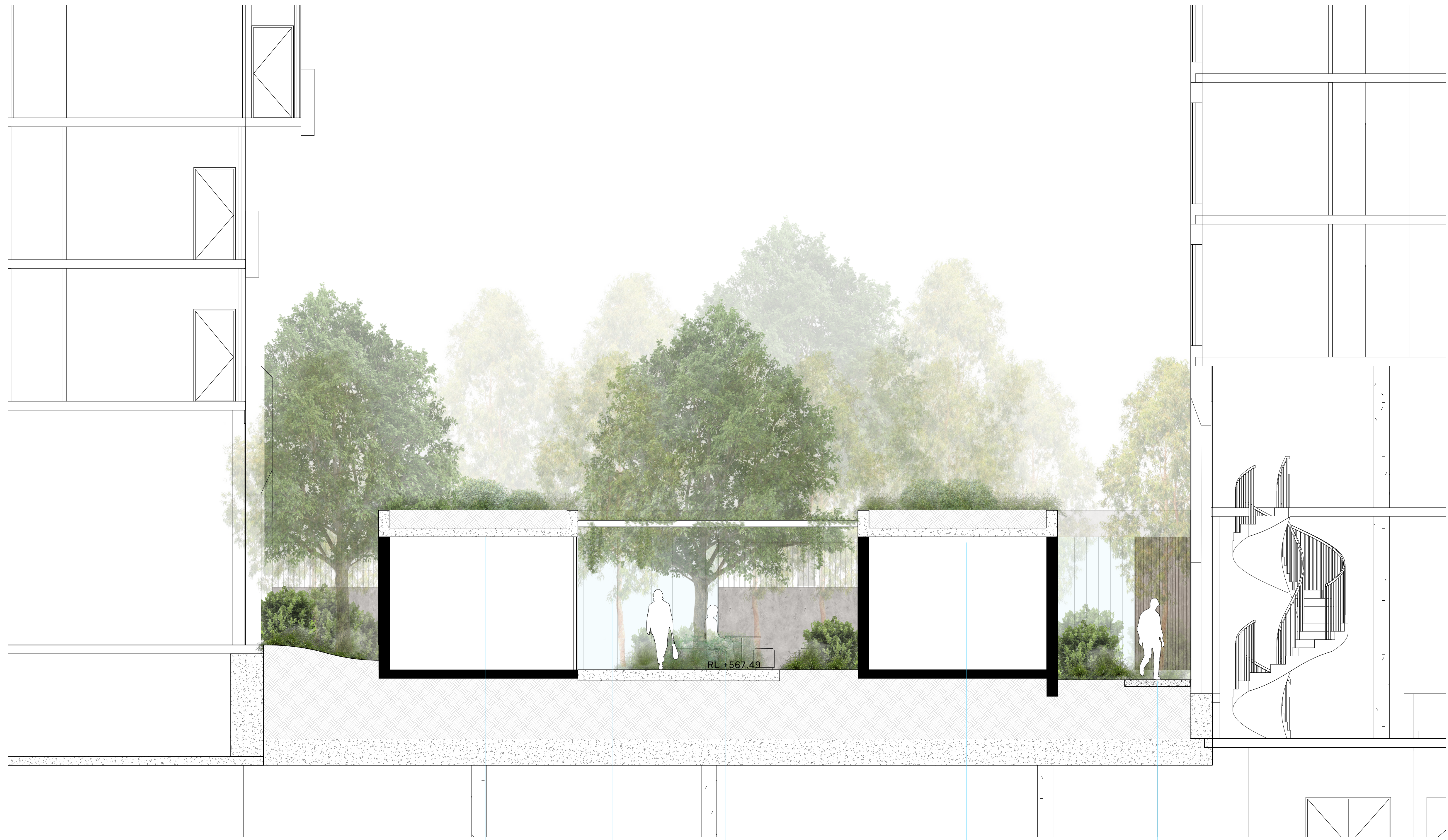
Section Elevation BB Scale: 1:50
