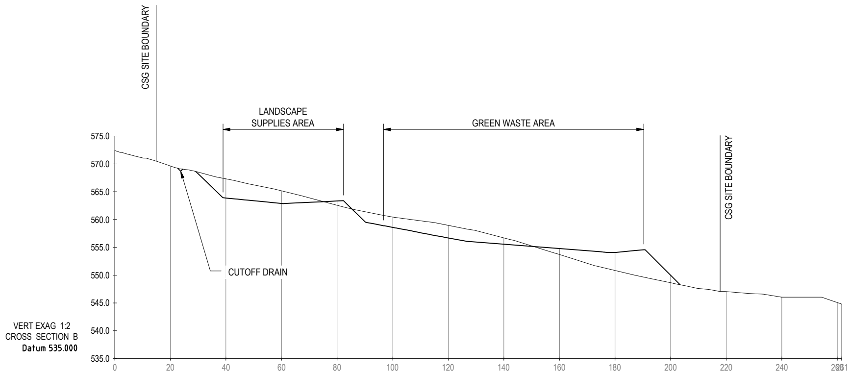
SECTION B D122
