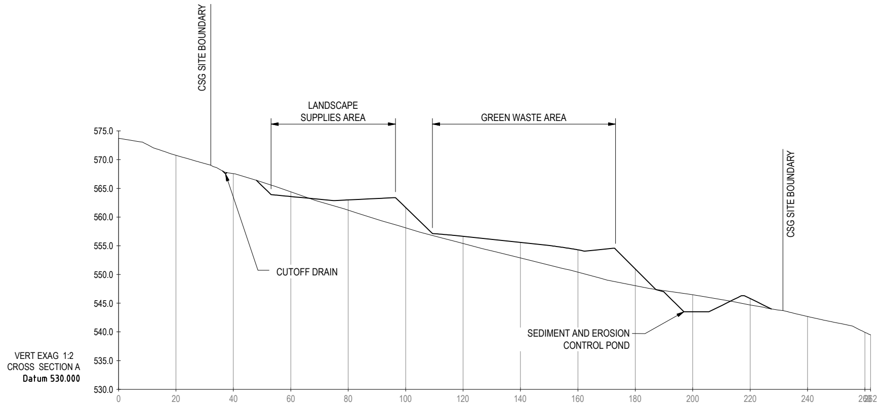
SECTION A D122
