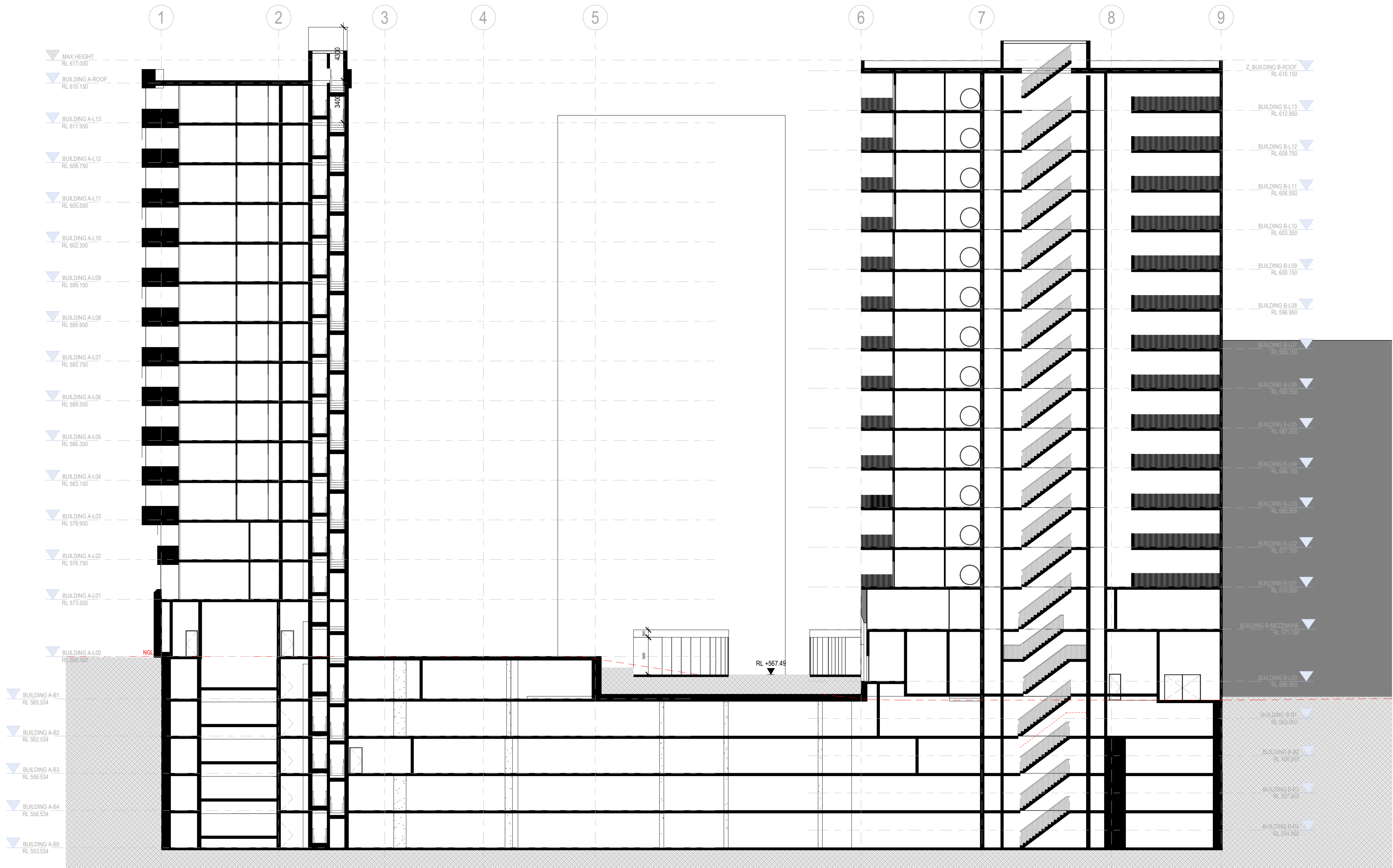
1 LONG SECTION 2 1 : 200
