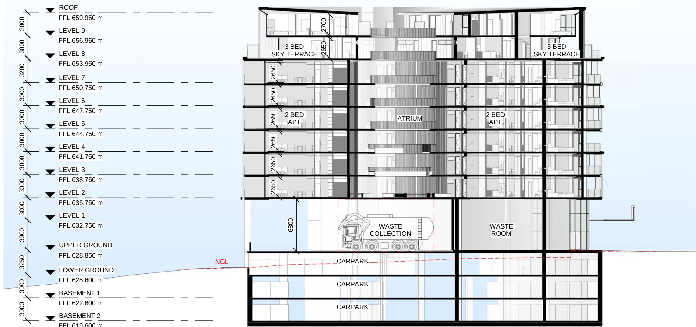
E SECTION E SCALE 1 : 300
