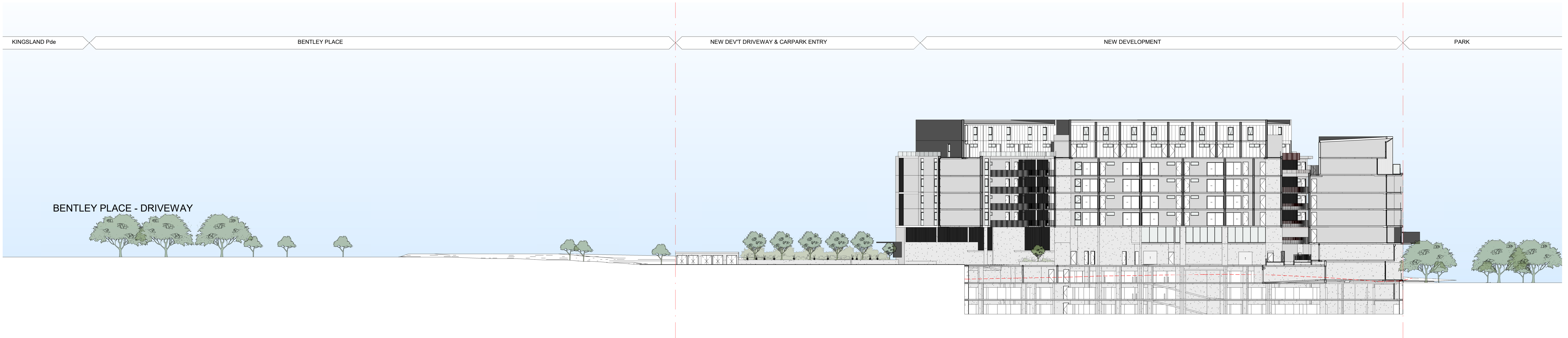
2 SITE SECTION B SCALE 1 : 350
