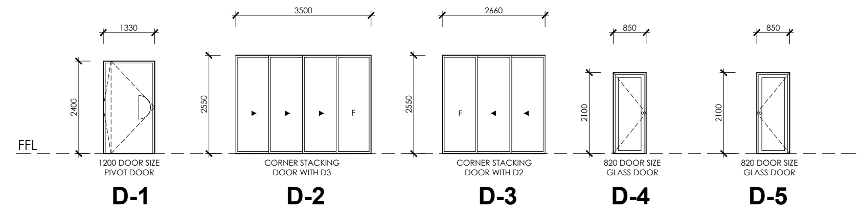
DOOR SCHEDULE
