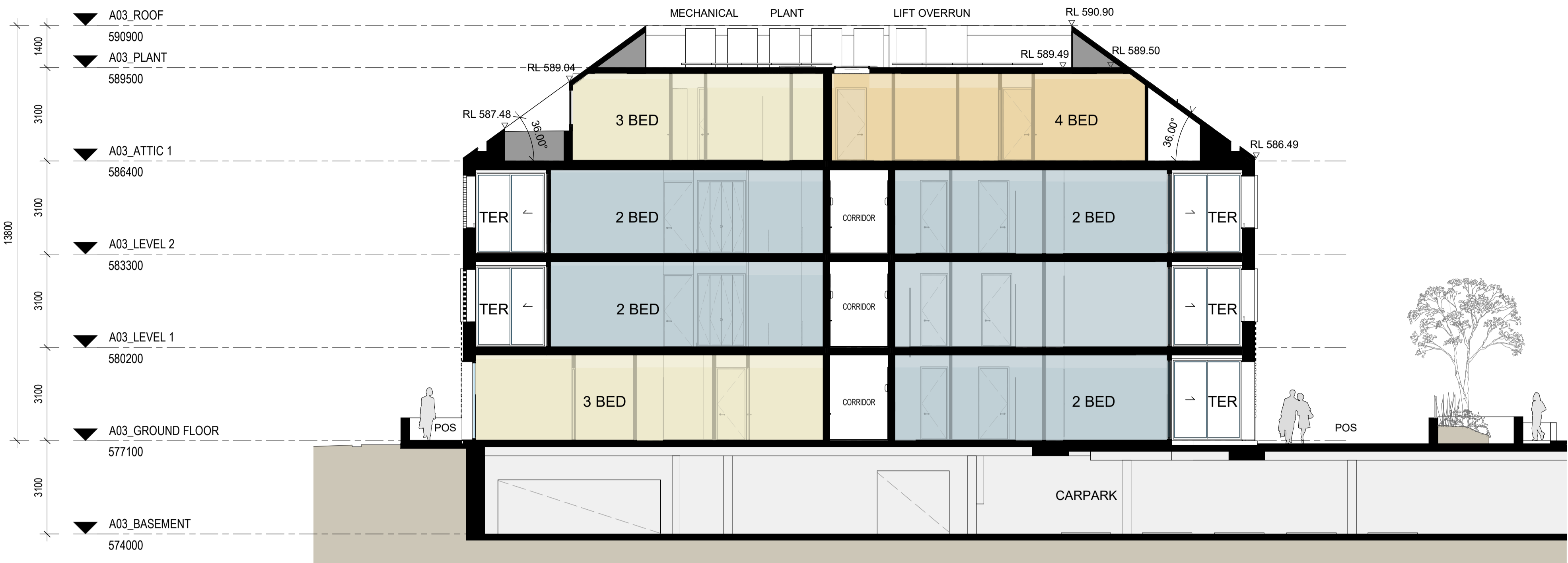
1 A03 - Section AA DA-A-0231 1:100@A1
