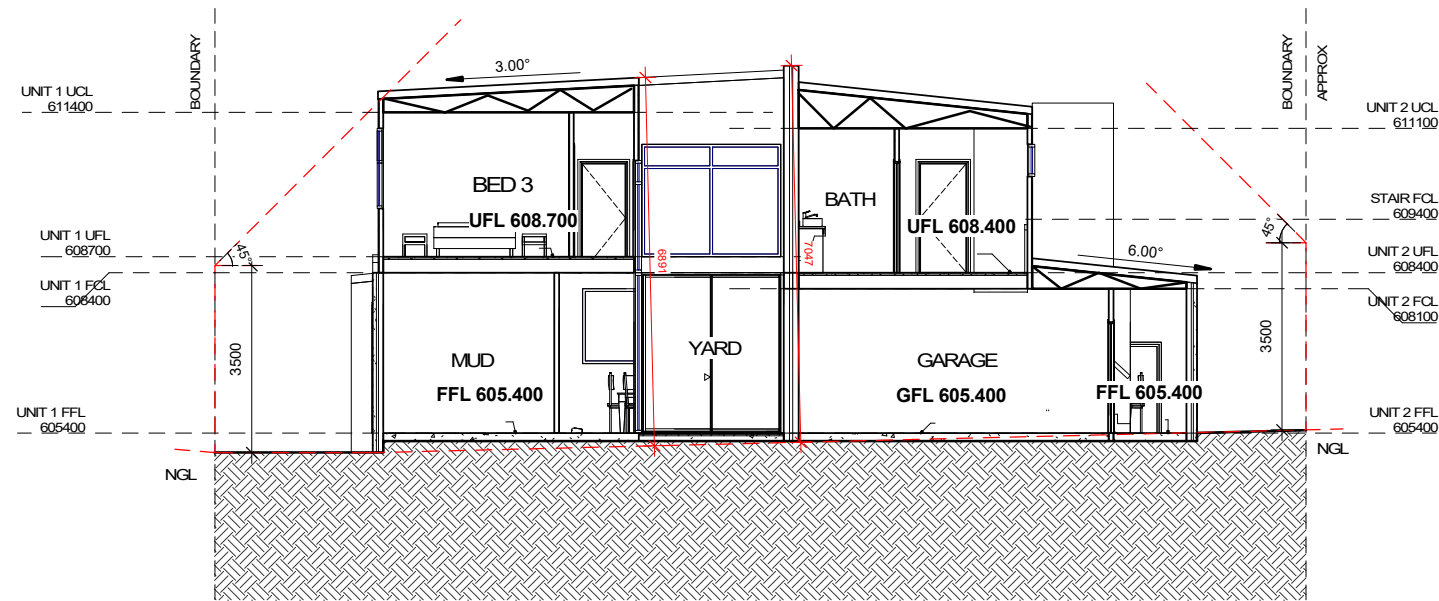
1 A 101 SECTION 1 : 100 unit 1 & 2 Section
