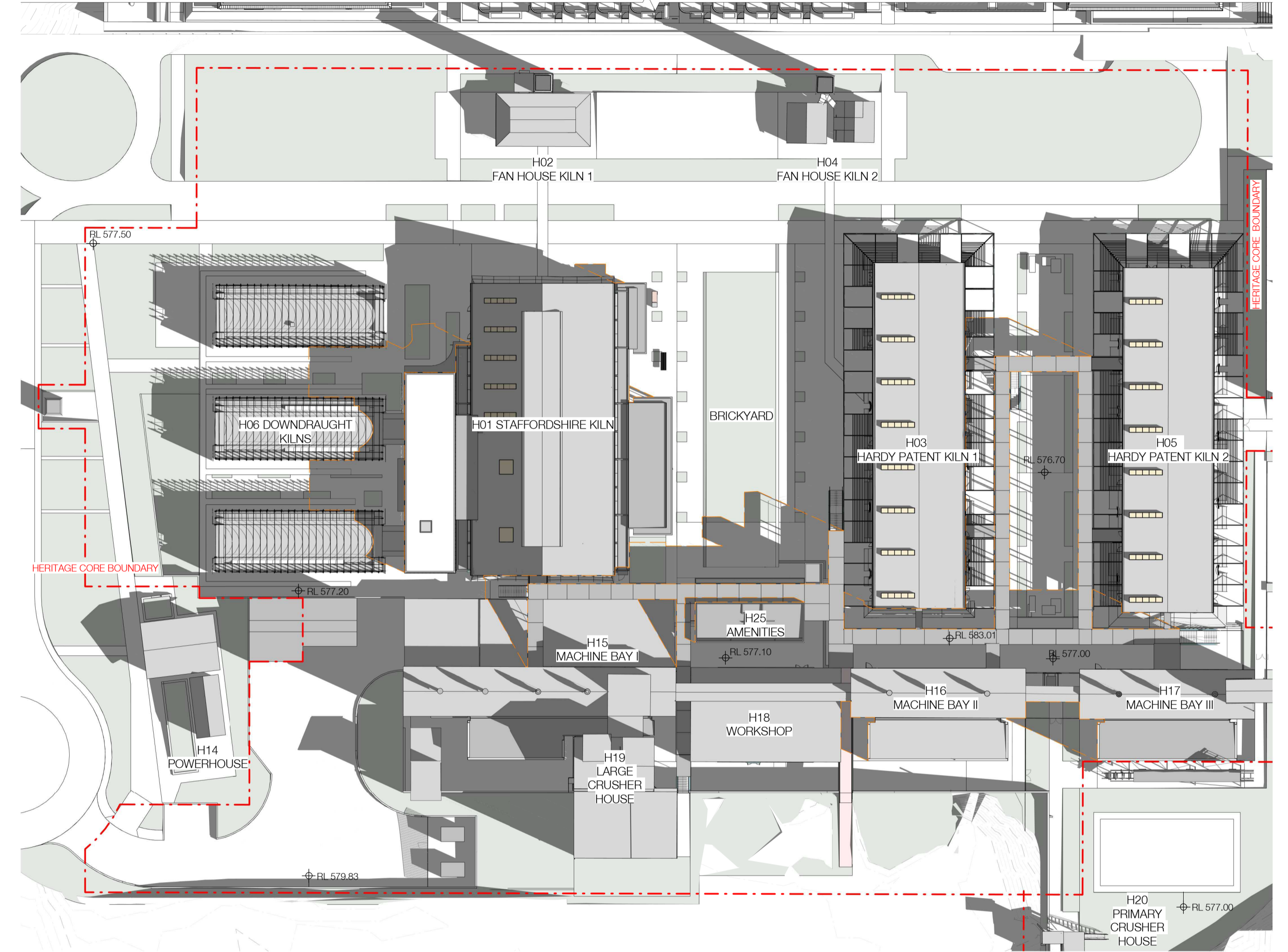
2 SHADOW PLAN - 21/06/2018-10.00 1: 500@A1
