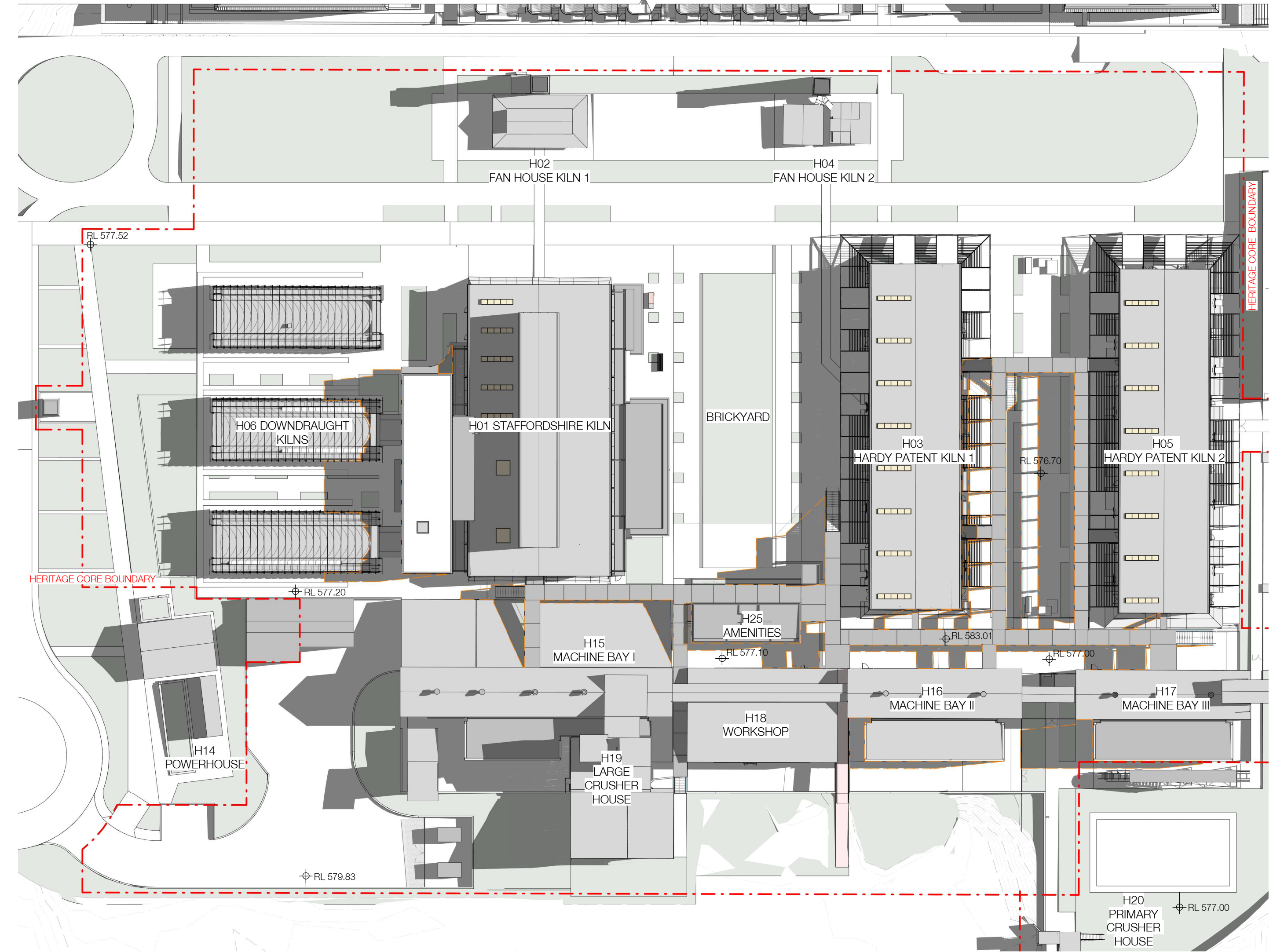
2 SHADOW PLAN - 21/06/2018-12.00 1 : 500@A1
