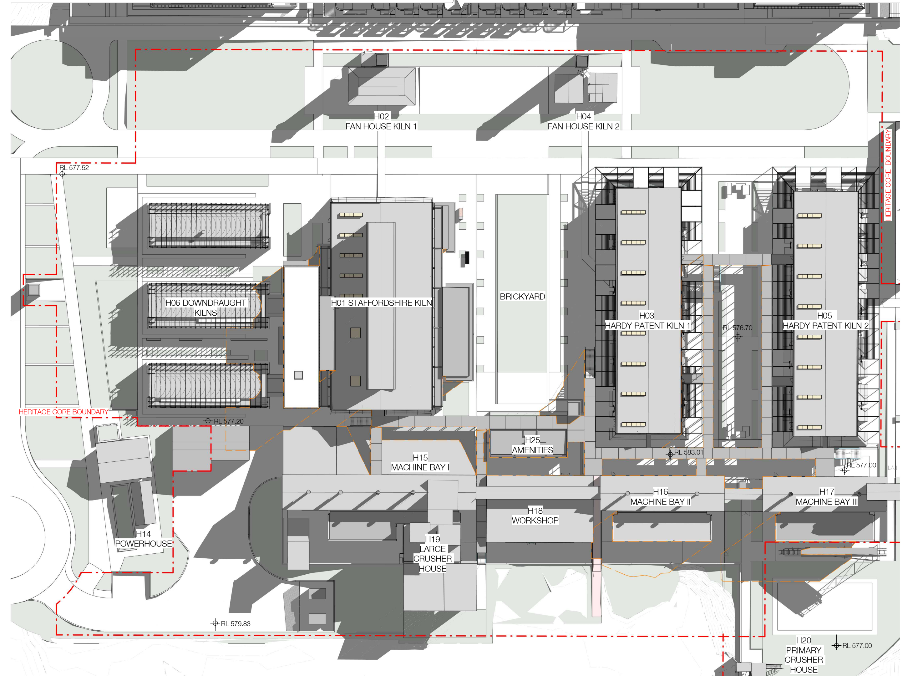
2 SHADOW PLAN - 21/06/2018-14.00 1 : 500@A1
