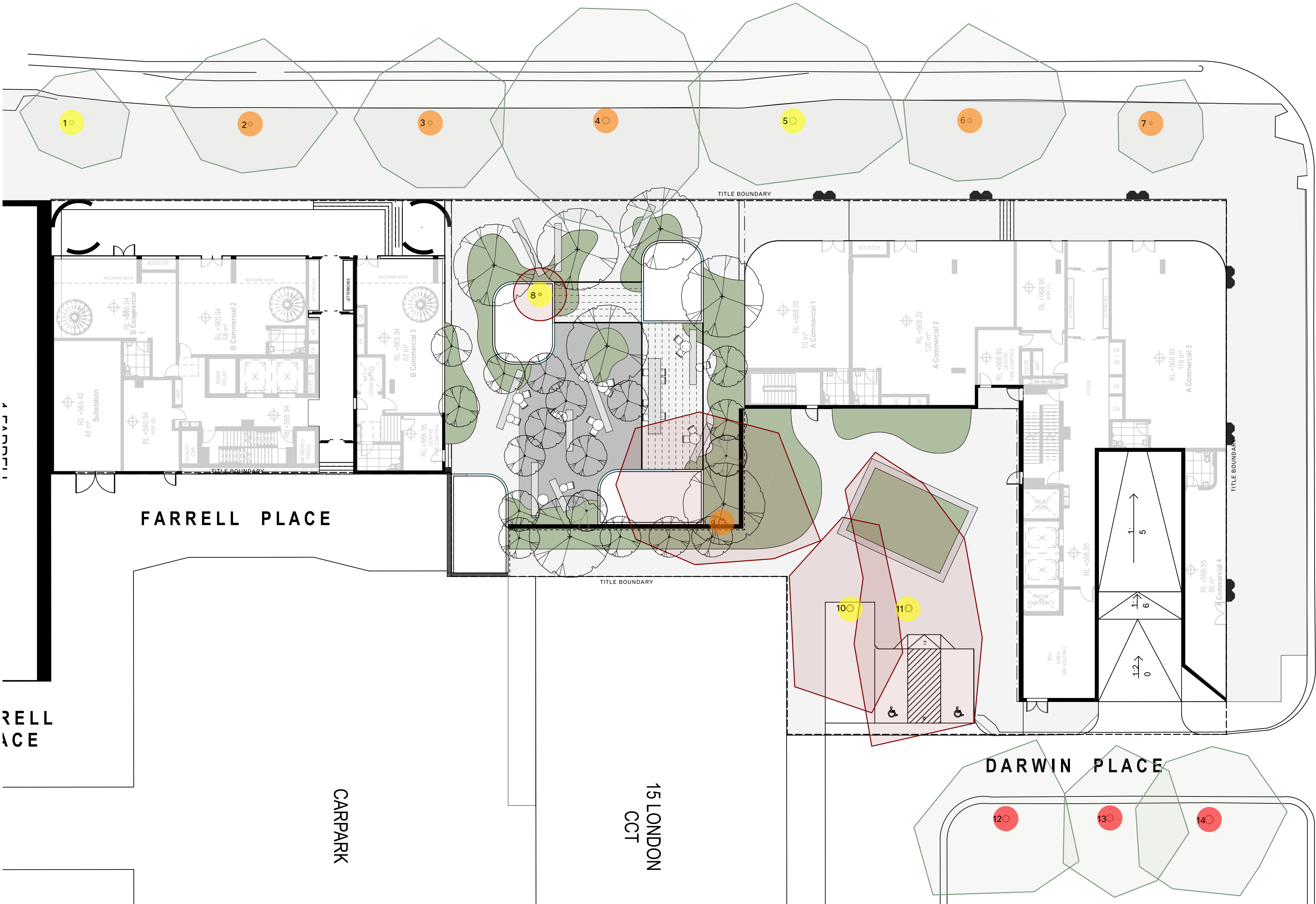
Landscape Plan Scale: 1:200
